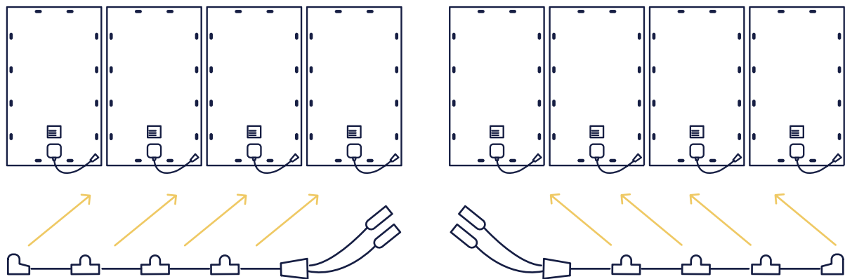
Vertikale Anbringung
