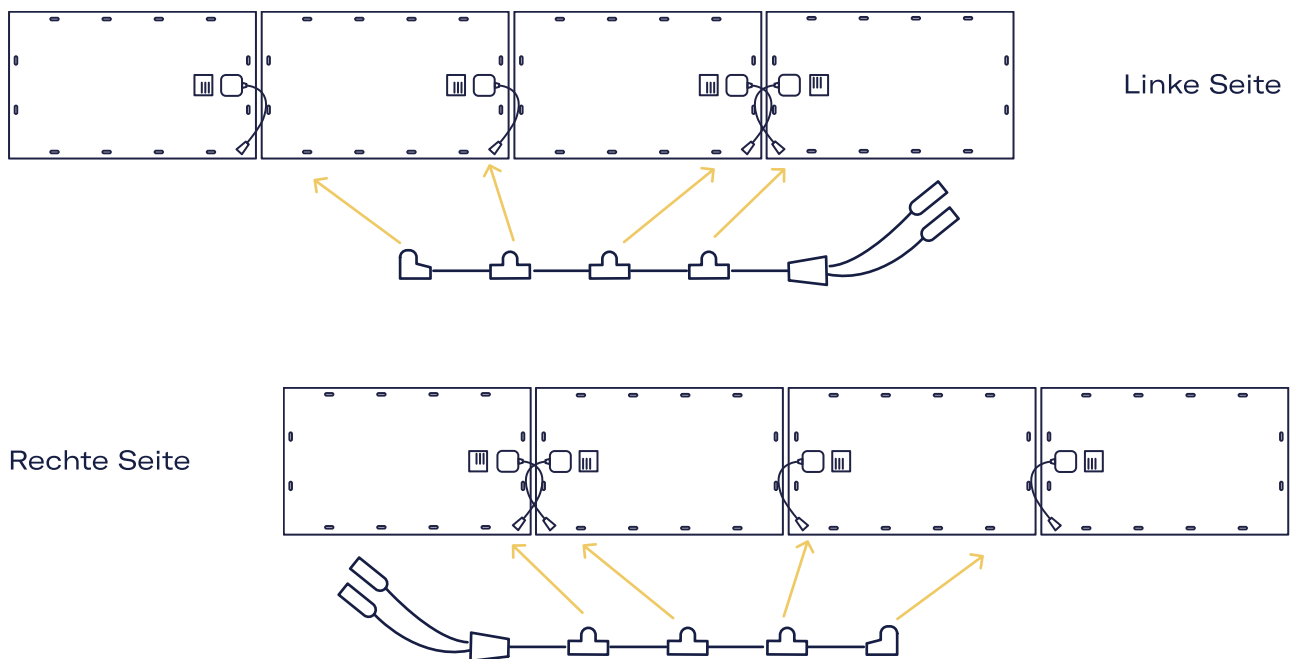
Horizontale Anbringung
