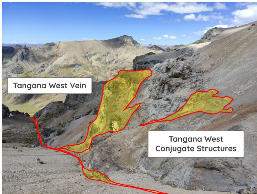
Abbildung 5: Regionale Ansicht des Erzgangs Tangana West und der mineralisierten konjugierten Strukturen.
