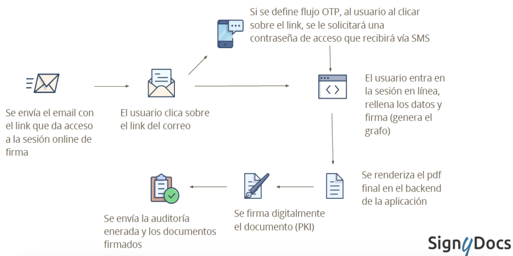
Figure 1 Flujo funcional de SignyDocs
