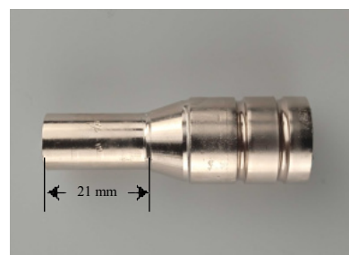
40600 Gasdüse zylindrisch, MR 14/15, NW10 flaschenform AD 12 mm/Länge: 21 mm Engspaltgasdüse
