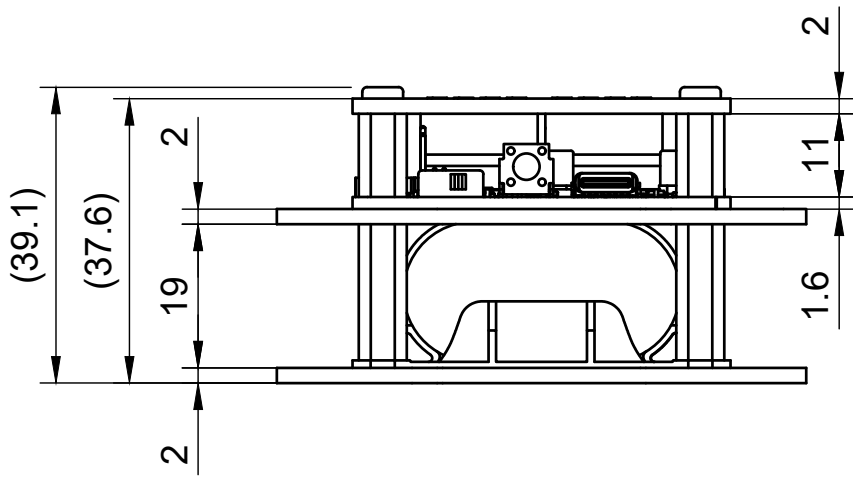
本体寸法図
