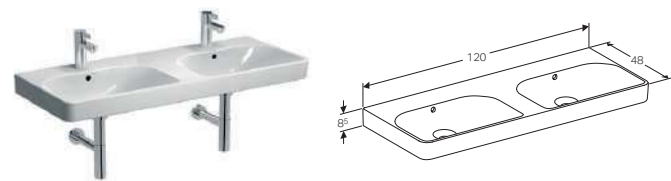
120cm square double washbasin W 120 / D 48 / H 8.5cm
