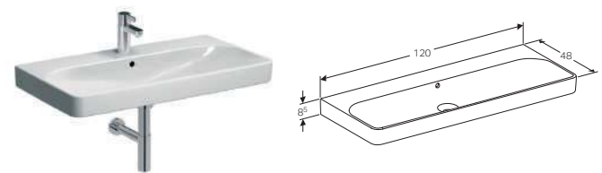
120cm square washbasin W 120 / D 48 / H 8.5cm
