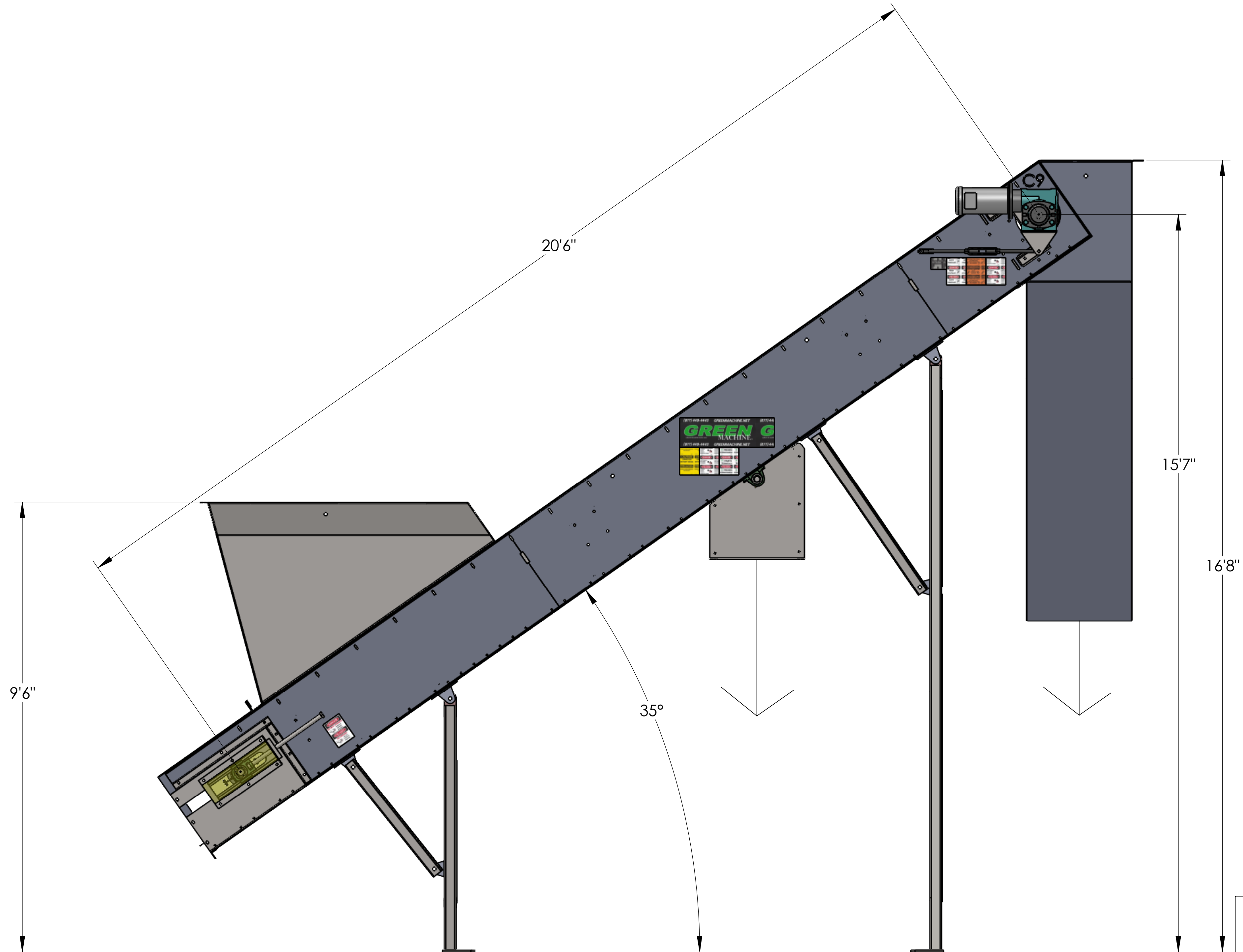
SECTION A-A
