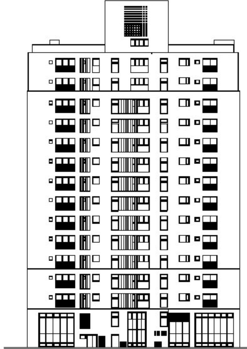
東向立面圖
