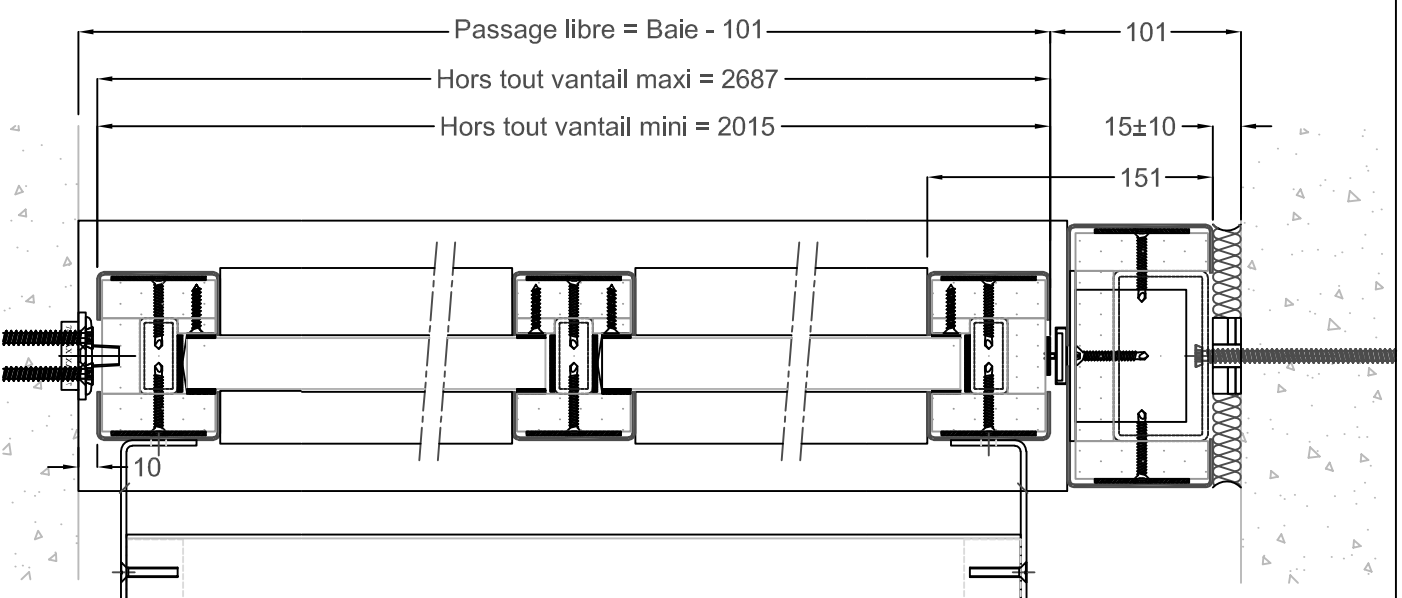
E30 - E/I30 - E/I60 Vitrage simple
