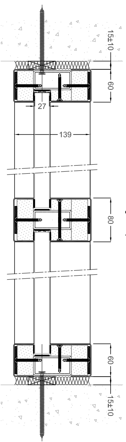
E30 - EI30 - EI60 Vitrage simple
