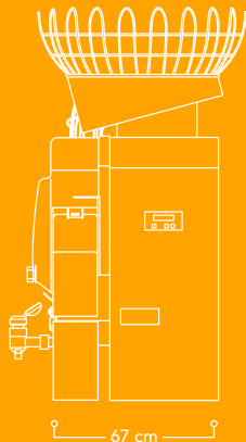
Seitenansicht
