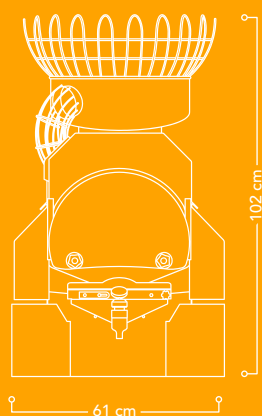
Vorderansicht
