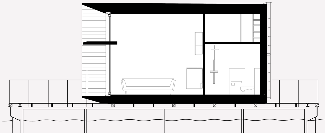
Coupe
