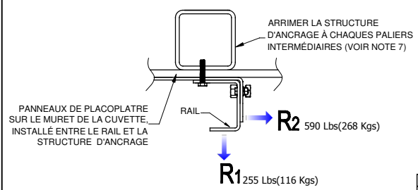
2 RÉACTIONS SUR RAIL
