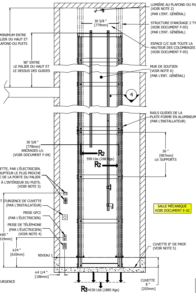
4 ÉLÉV. DU MUR DE SOUTIEN
