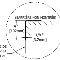
7 DÉTAIL C SEUIL DE BARRIÈRE
