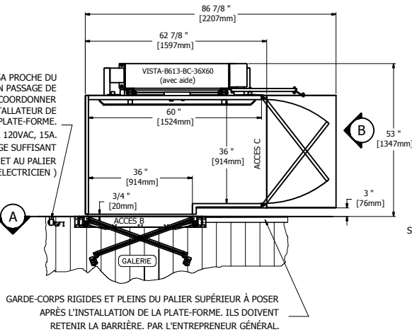
1 VISTA-613-BC 36x60 AVEC AIDE
