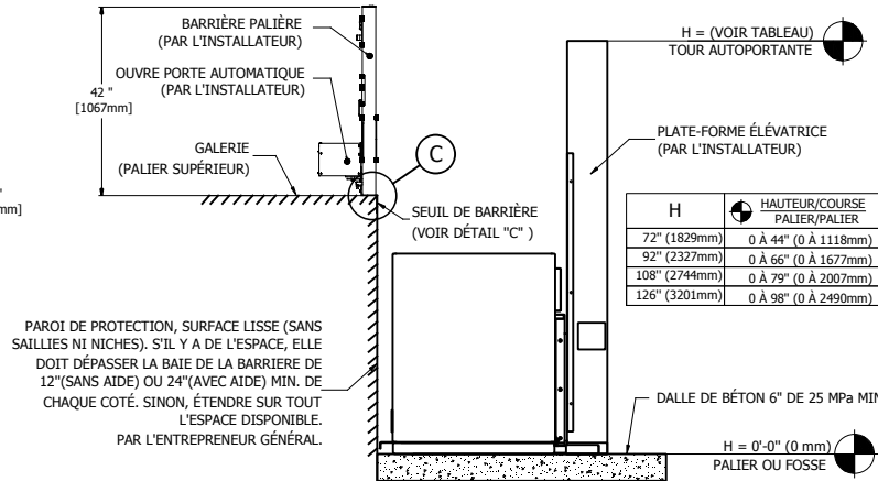
2 DÉTAIL A VUE DE FACE
