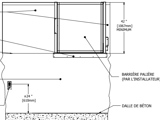
3 DÉTAIL B VUE DE CÔTÉ
