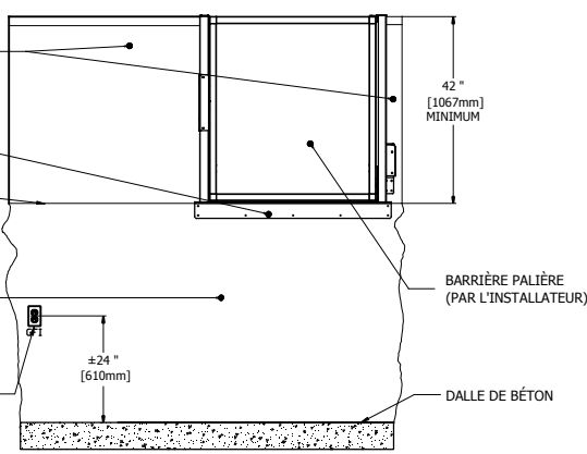
3 DÉTAIL B VUE DE CÔTÉ
