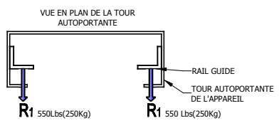
4 RÉACTIONS SUR RAIL
