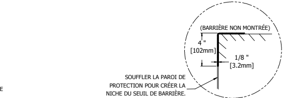
7 DÉTAIL C SEUIL DE BARRIÈRE
