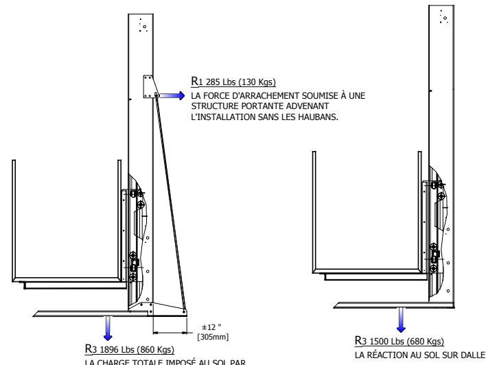
5 VISTA-1000 Lbs RÉACTIONS
