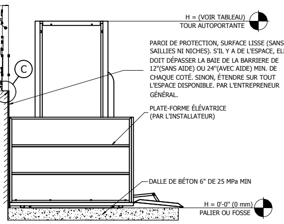
2 DÉTAIL B VUE DE FACE
