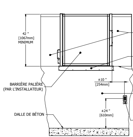
3 COUPE A VUE DE CÔTÉ
