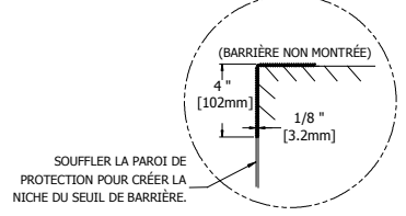
7 DÉTAIL C SEUIL DE BARRIÈRE
