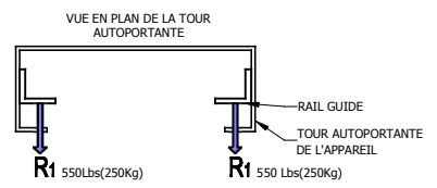
RÉACTIONS SUR RAIL
