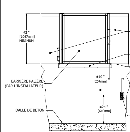
3 COUPE A VUE DE CÔTÉ
