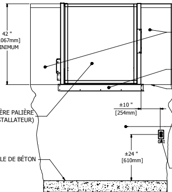
3 COUPE A VUE DE CÔTÉ
