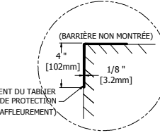
7 DÉTAIL "C" SEUIL DE BARRIÈRE
