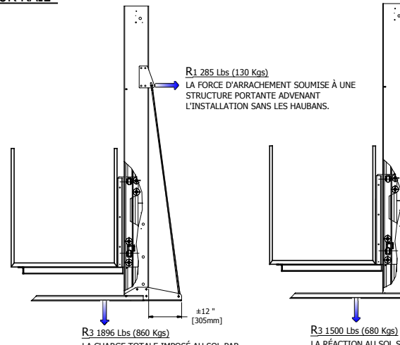
5 VISTA 1000 Lbs RÉACTIONS
