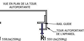
4 RÉACTIONS SUR RAIL
