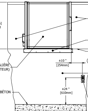
3 COUPE A VUE DE CÔTÉ
