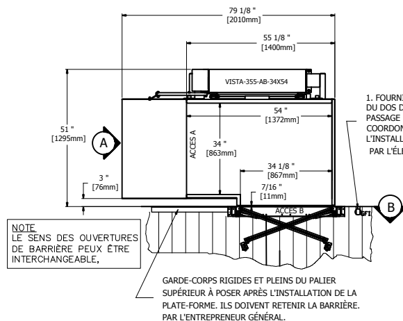
1 VISTA-355-AB 34x54 SANS AIDE
