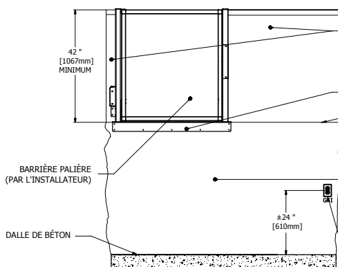
3 COUPE B VUE DE CÔTÉ
