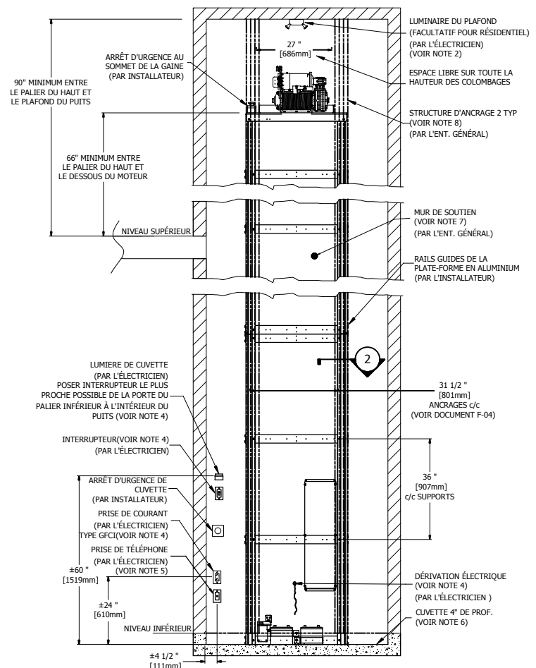
4 ÉLÉV. DU MUR DE SOUTIEN
