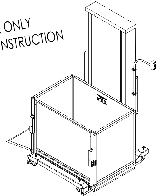
VUE ISOMÉTRIQUE
