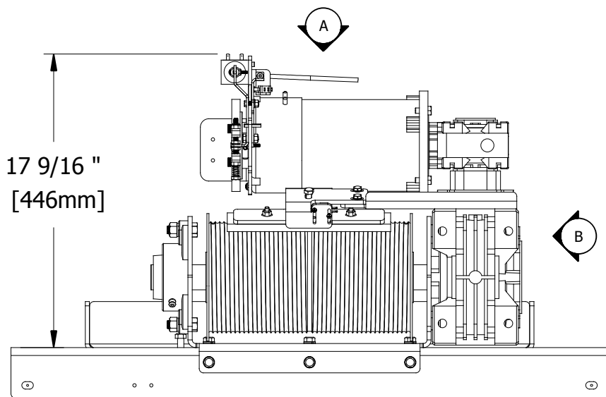
DÉTAIL C ELEVATION
