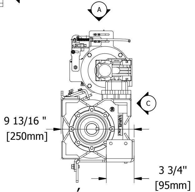
DÉTAIL B SIDE VIEW
