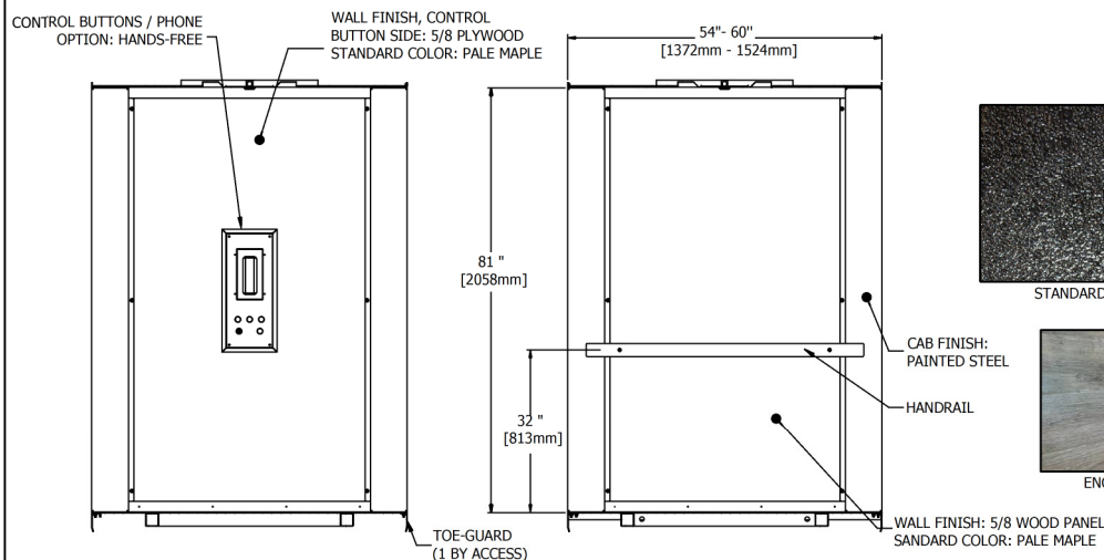
ELEVATION A
