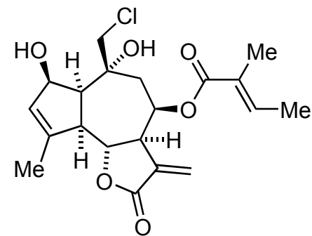
Eupalinilide E
