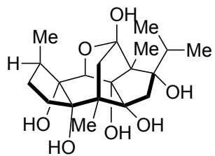
(+)-perseanol
