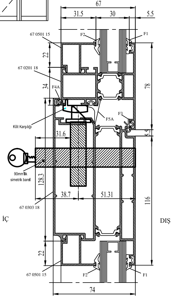
DETAY 4
