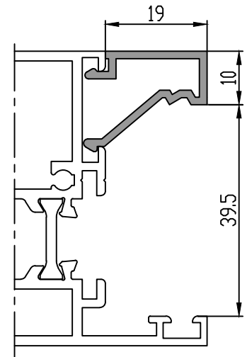
55 0502 14: 0.241 kg/m
