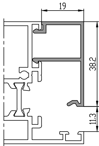
51 5007 14: 0.356 kg/m 51 5007 20: 0.479 kg/m
