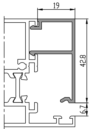
51 5065 15: 0.396 kg/m
