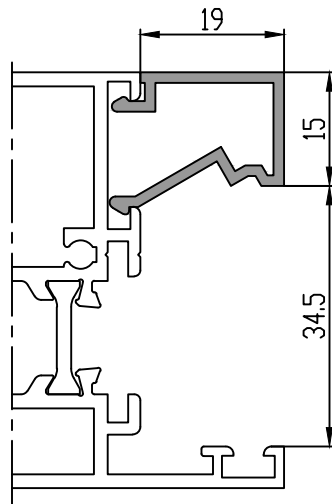
51 5039 14: 0.259 kg/m
