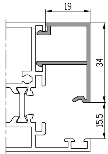
51 5006 10: 0.248 kg/m 51 5006 14: 0.340 kg/m
