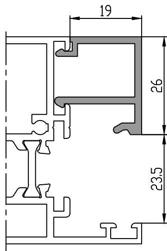
51 5042 12: 0.267 kg/m 51 5042 18: 0.381 kg/m
