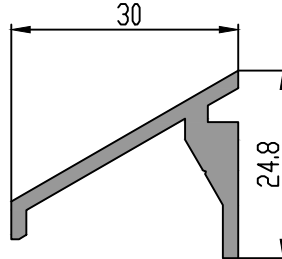
Damlalık Profili
