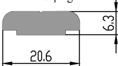
Kilit Karşılığı
