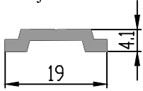
Tij Profili
