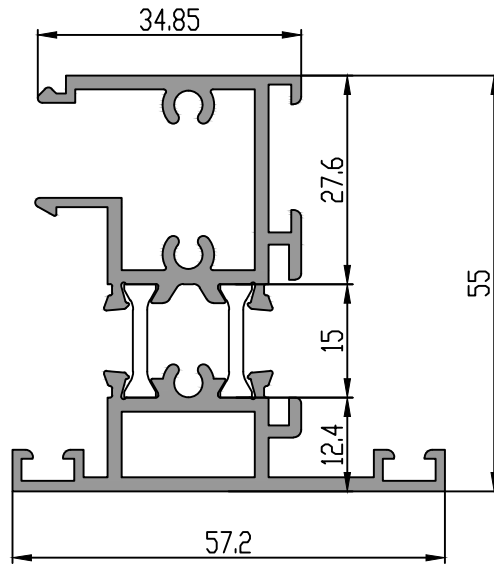
Çift Kanat Adaptörü
