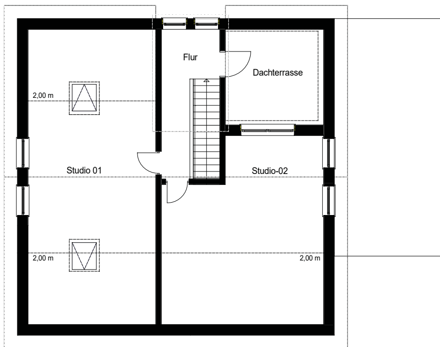
T04-03-Dachgeschoss
